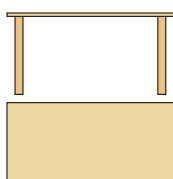
Mesa auxiliar de centro 125 x 60 x 61 H cm
