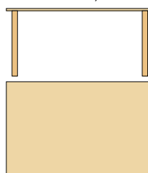
Mesa de comedor 160 x 85 x 75,5 H cm
