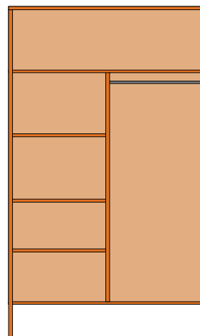
ARB-90-02 90 x 60 x 200 H cm ARB-120-02 120 x 60 x 200 H cm
